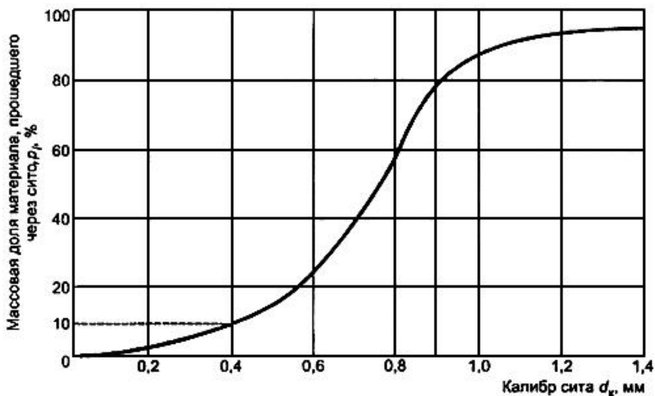
Рисунок А.1 - График ситового анализа материала
